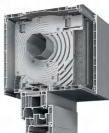
Durchgängiges Statikkonzept
